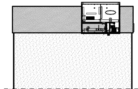
Plattegrond tweede verdieping
